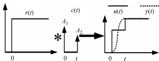
图 4 输入整形原理图
