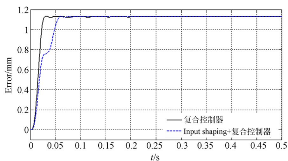
图 9 运动平台的实际响应曲线
