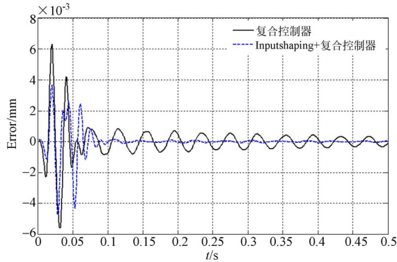
图 10 运动平台的位置误差曲线
