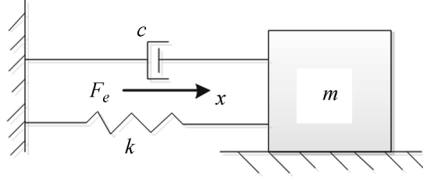
图 1 运动平台力学模型
