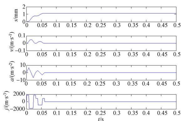
图 7 输入整形后的三阶输入轨迹
