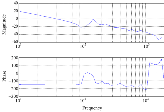
(c) 频域响应
