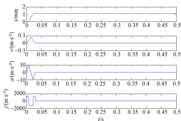
图 6 三阶输入轨迹
