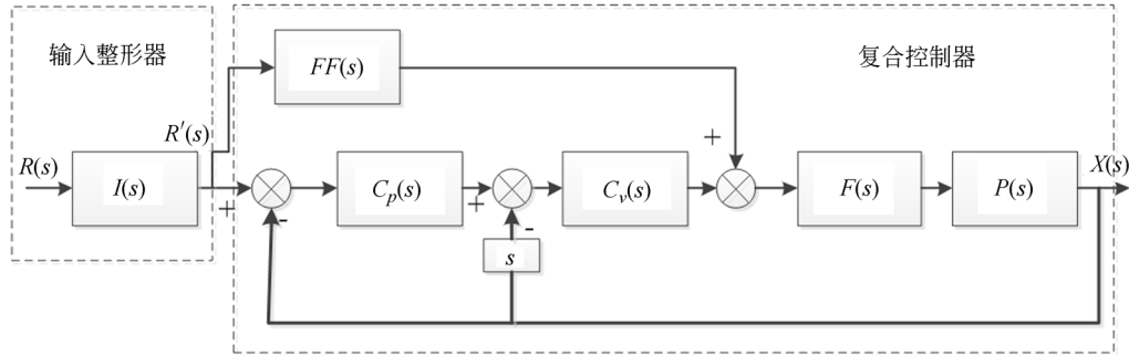
图 5 运动平台控制系统结构图
