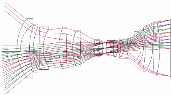
图 5 光学系统结构图
