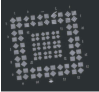
图11 相机对IV号鉴别率板成像照片
