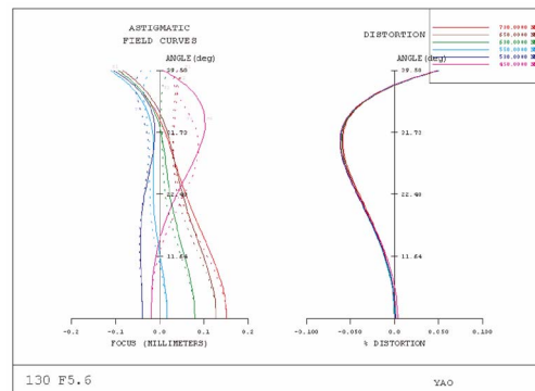
图 8 光学系统场曲与畸变曲线
