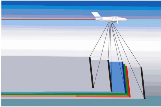
图 4 大视场三线阵航空测绘相机工作原理图
