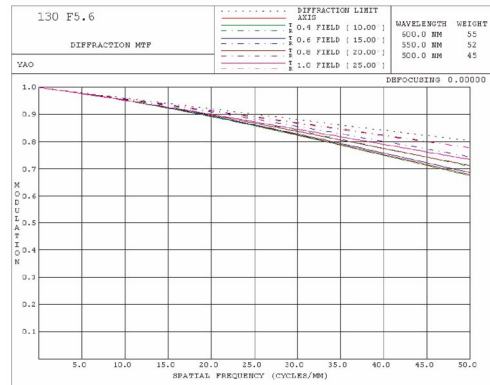
(b)G 谱段调制传递函数曲线
