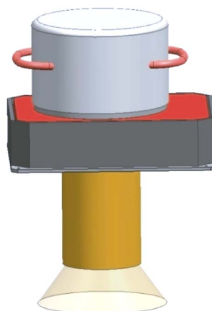
图 2 单镜头方案相机模型图
