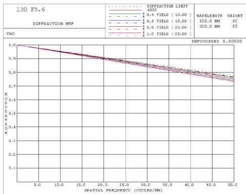
(a)R 谱段调制传递函数曲线
