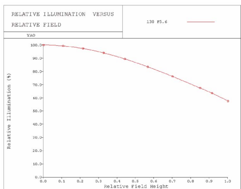
图 9 光学系统相对照度曲线
