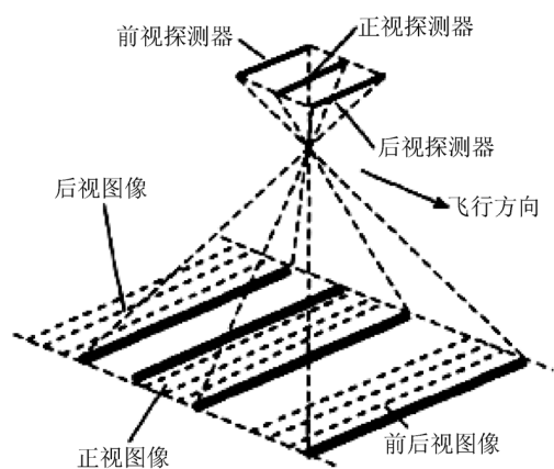
图 1 三线阵相机测绘原理图
