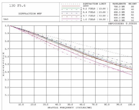
图 6 光学系统全色谱段调制传递函数曲线
