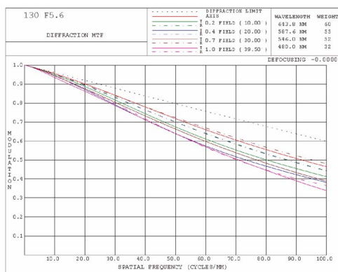
(b)0 °C 时调制传递函数曲线
