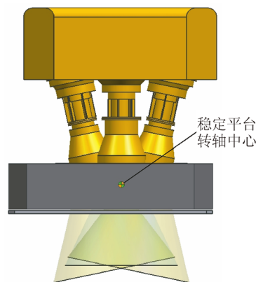
图 3 三镜头拼接方案相机模型图
