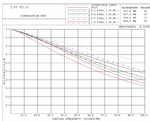
(c)40 °C 时调制传递函数曲线
