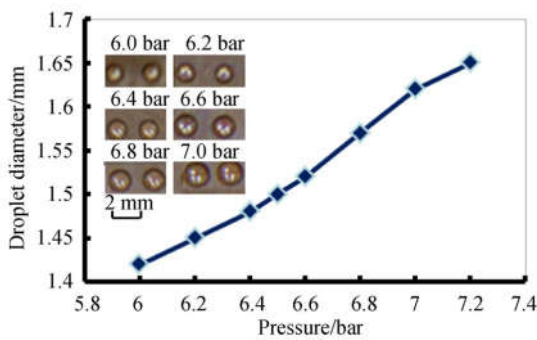
图 11 胶点直径与供胶压力关系图
