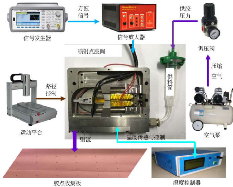
图 10 点胶阀性能测试系统
