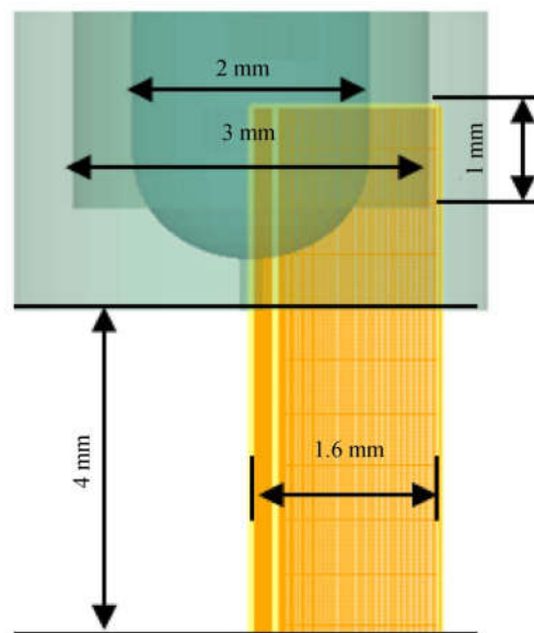
图 6 仿真流体模型 Fig. 6 Fluid model in Simulation
