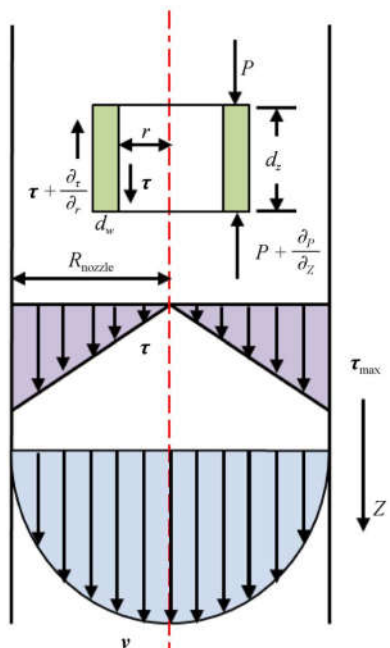
图 5 胶体微元动力学分析示意图 Fig. 5 Schematic diagram of colloidal micro-element dynamics analysis
