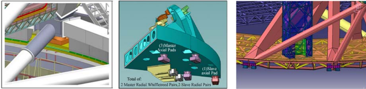
(a)TMT 望远镜六个方位轴静液压油垫之一 (b)GMT 望远镜方位轴 1/4 基座底部静液压油垫 (c)E-ELT 望远镜的方位轴静液压油垫系统
