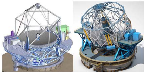
(a)三十米望远镜 (a)TMT
