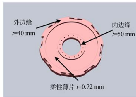
图 5 中心膜片(殷钢)
