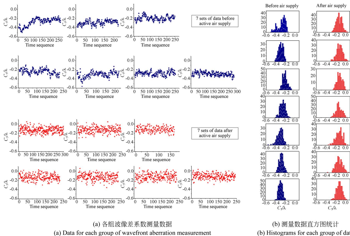
图 7 主动送风前后 7 组波像差系数测量数据及其直方图
