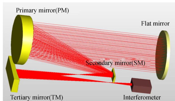
图 1 自准直干涉光路示意图
