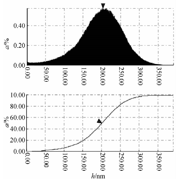
图 6 电极表面形貌高度比例图和高度直方图
