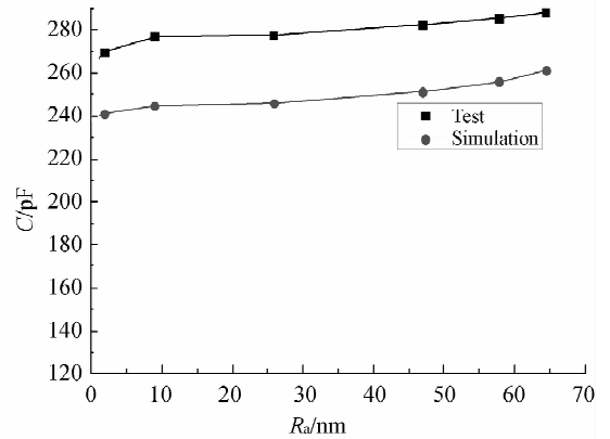
图 7 不同表面平均粗糙度对检测电容的影响
