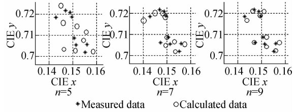
图 8 绿光 LED 的测量色坐标与计算色坐标
