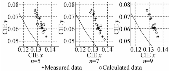
图 7 蓝光 LED 的测量色坐标与计算色坐标
