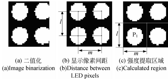
图 4 LED 显示像素点的强度值提取区域
