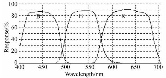
图 6 理想状态的光谱响应函数
