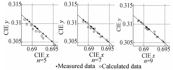
图 9 红光 LED 的测量色坐标与计算色坐标
