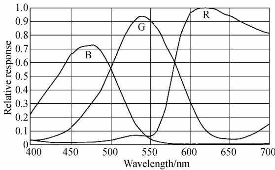
图 5 彩色 CCD 相机的光谱响应函数
