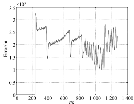
图 9 弹道预测误差
