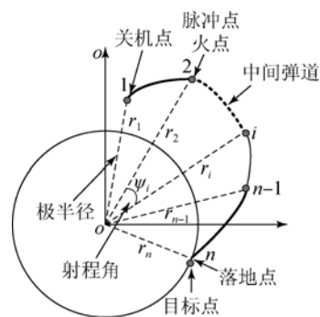
图 1 单脉冲变轨示意图
