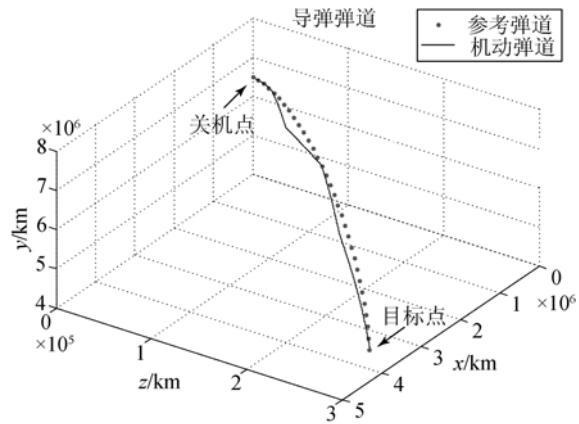
图 7 变轨弹道仿真示意图
