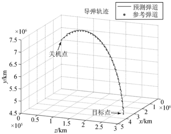
图 10 参考弹道预测示意图
