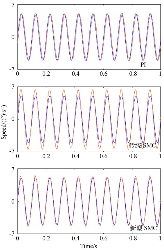
图 3 正弦波跟踪曲线 Fig. 3 Tracking curves of sine wave
