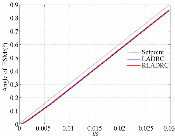
图 8 FSM 斜坡响应曲线
