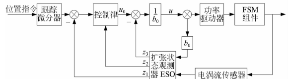
图 3 FSM 通用自抗扰控制器
