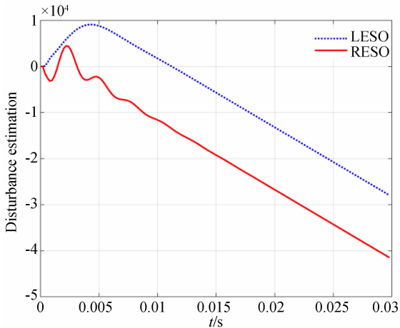
图 9 斜坡响应 LESO 和 RESO 的扰动估计值
