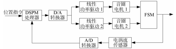
图 5 FSM 控制原理图
