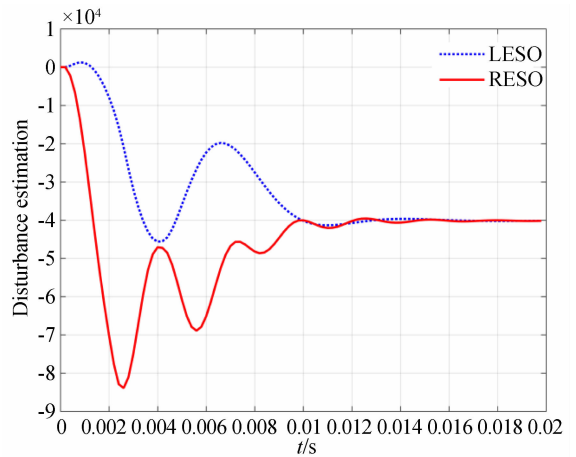
图 7 阶跃响应 LESO 和 RESO 的扰动估计值
