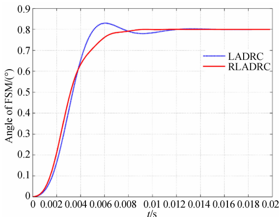
图 6 FSM 阶跃响应曲线
