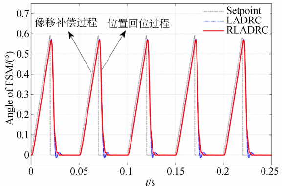
图 12 FSM 连续工作曲线
