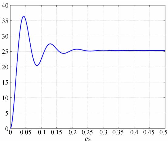
图2 FSM 开环阶跃响应曲线
