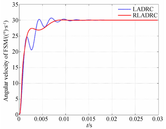
图 11 FSM 斜坡响应速度曲线
