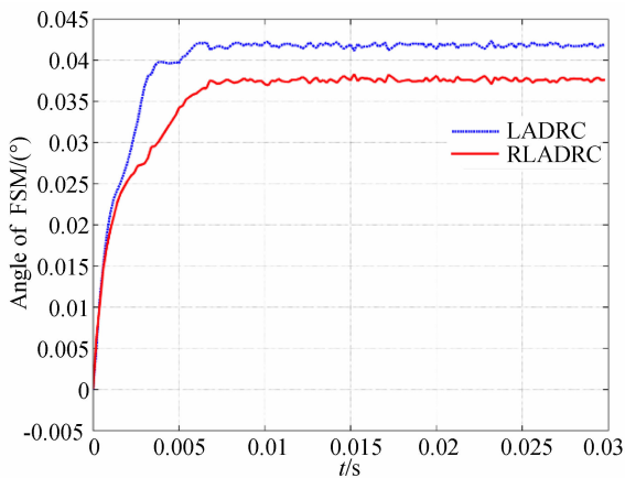
图 10 FSM 斜坡响应位置误差曲线
