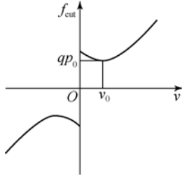
图 2 干摩擦特性曲线
