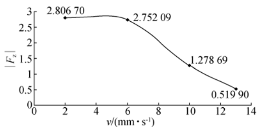
图 5 刻划速度 v 对 F_z 的影响
