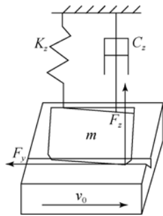
图 3 摩擦型颤振系统动力学模型
