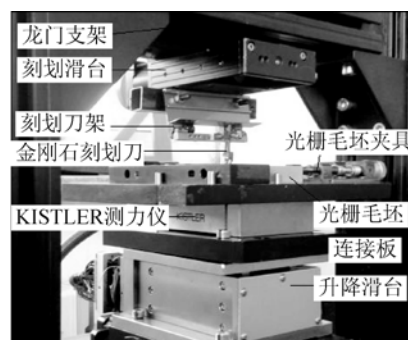
图 4 光栅机械刻划工艺试验装置
