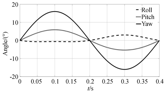
图 3 负载姿态角度的变化曲线
