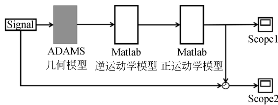
图 5 逆运动学仿真系统
