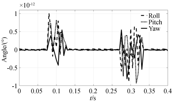
图 4 姿态角输出误差
