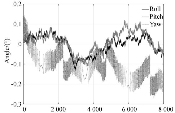
图 11 负载角度误差 Fig. 11 Load angle errors
