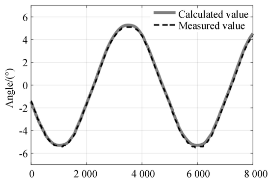
图 10 负载的方位角度 Fig. 10 Yaw angle of load
