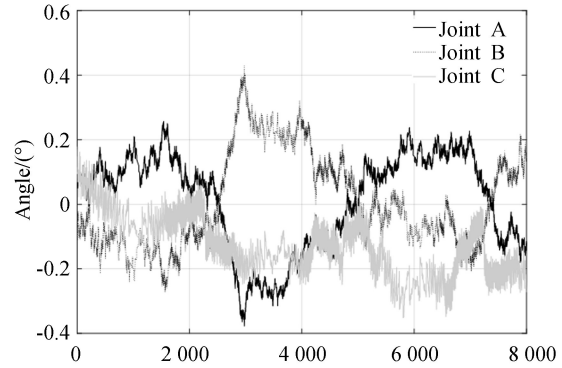
图 15 转动副的角度误差
