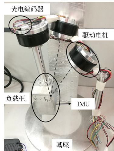
图 7 串联球面机构运动学验证装置
