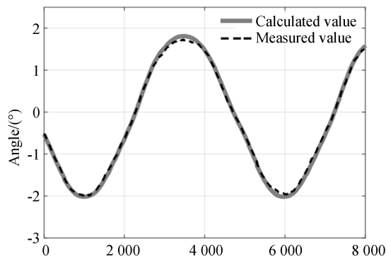
图 9 负载的俯仰角度 Fig. 9 Pitch angle of load
