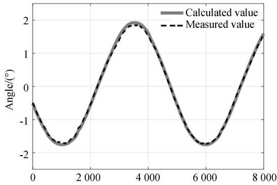
图 8 负载的滚转角度 Fig. 8 Roll angle of load
