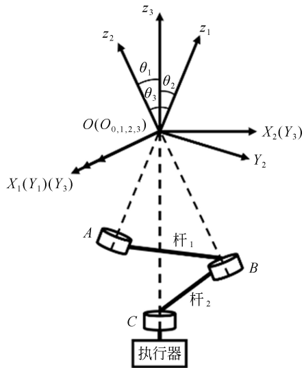
图 1 串联球面机构坐标系示意图
