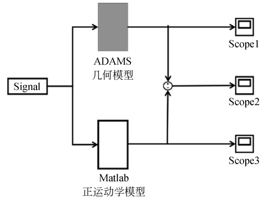
图 2 正运动学联合仿真验证
