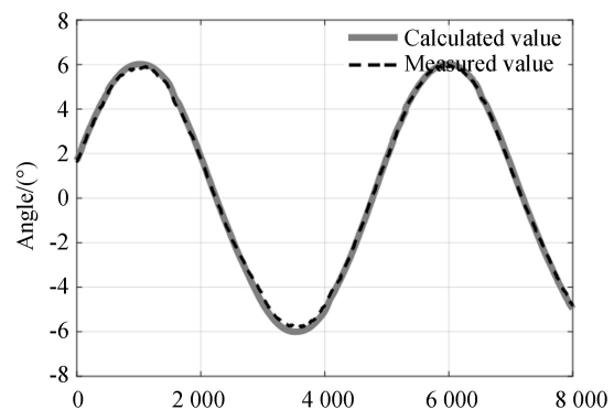
图 12 转动副 A 的角度 Fig. 12 Angle of revolute joint A
