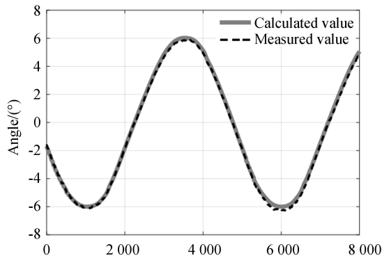
图 14 转动副 C 的角度
