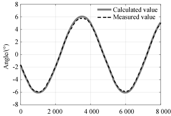
图 13 转动副 B 的角度
